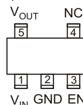
SOT-353 (SC-70-5L)
