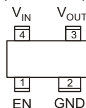
SOT-343 (SC-70-4L)
